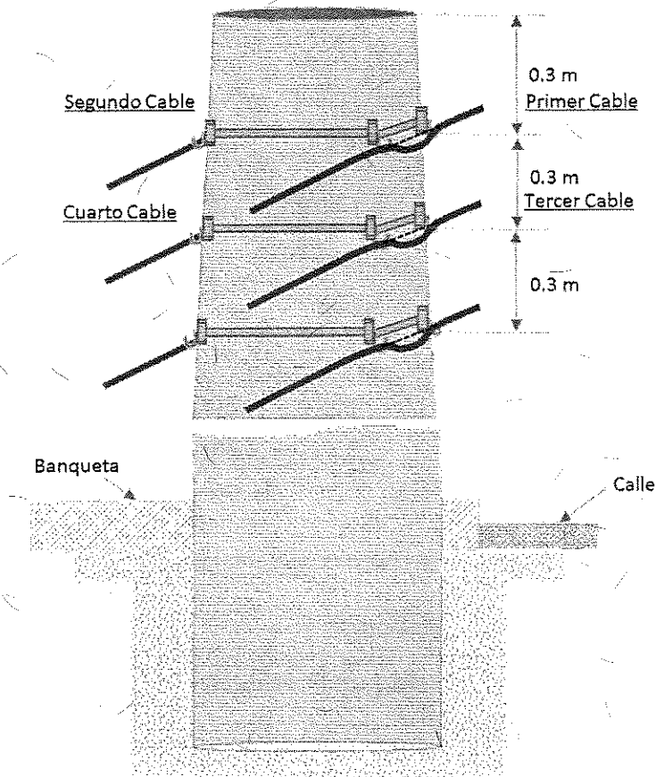
Figura 10. Ordenamiento de cableado en Poste
