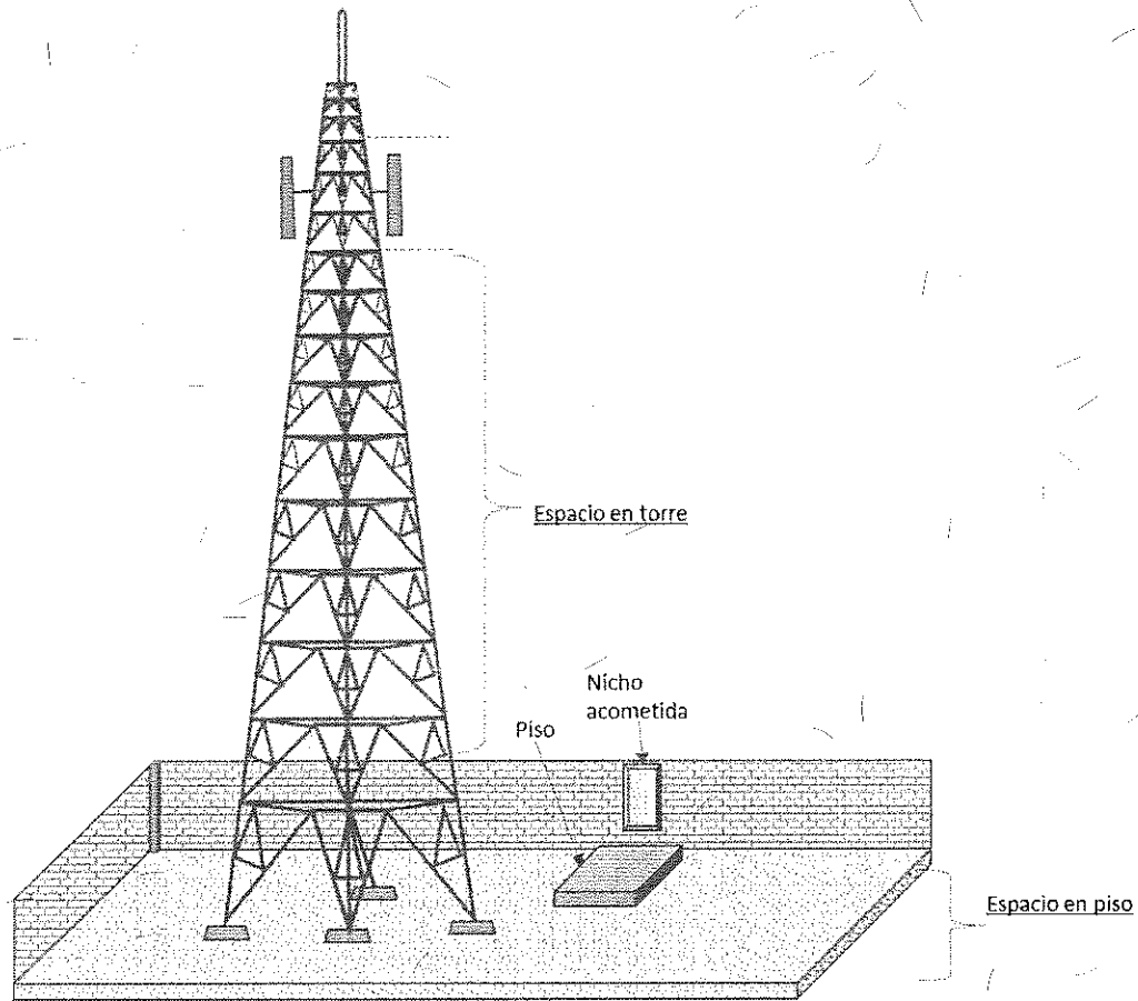
Figura 6. Espacio de compartición
