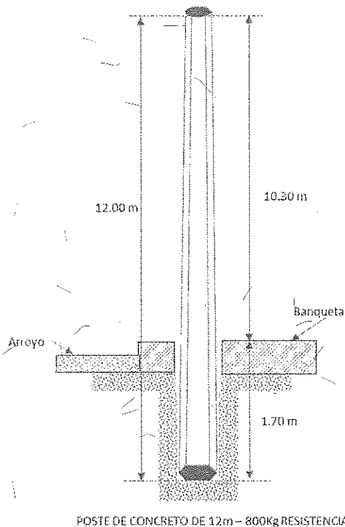
POSTE DE CONCRETO DE 12m - 800Kg RESISTENCIA
