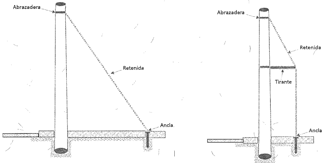
Figura 5. Retenida en Poste
