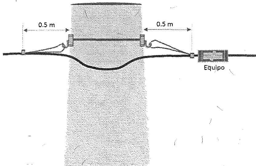
Figura 6. Libramiento de equipo/accesorios en Poste
