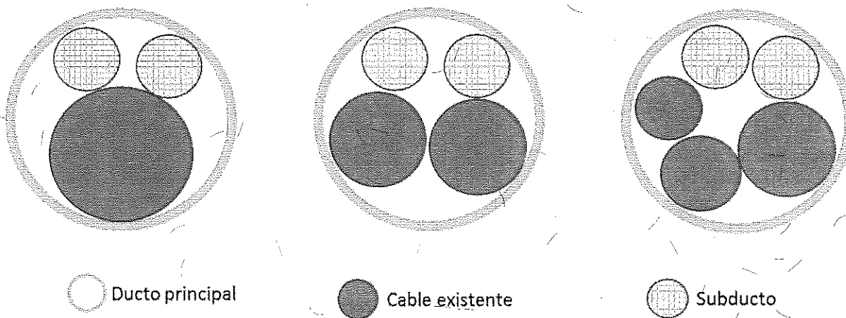
Figura 8. Ejemplos de subductos en Ducto principal con cables existentes
