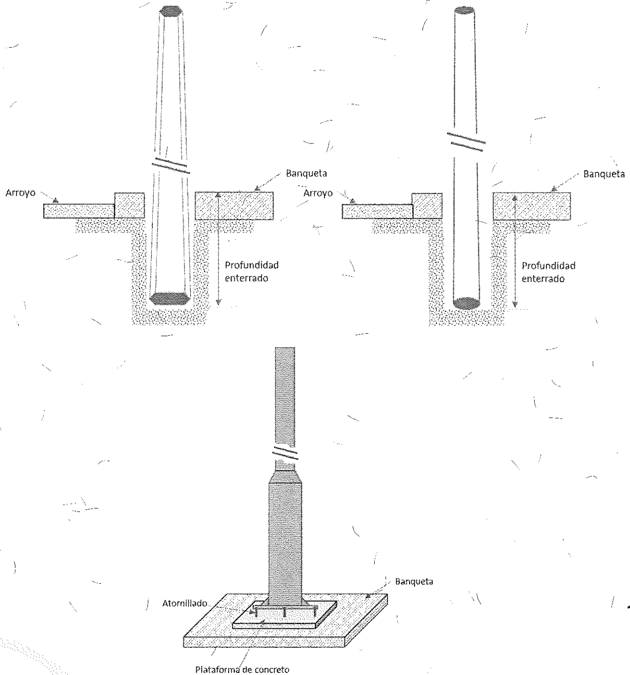
Figura 2. Instalación de Poste de concreto, madera y acero
