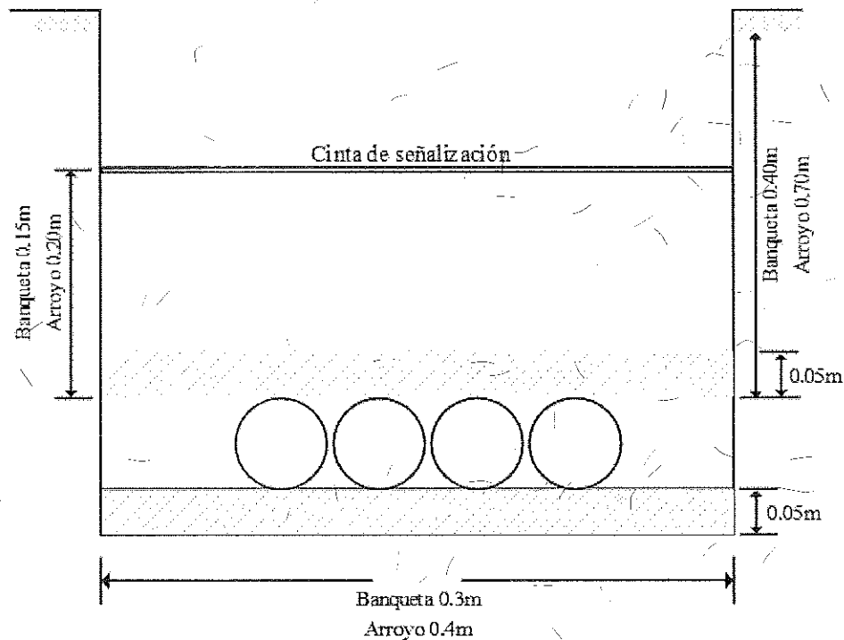
Figura 1. Esquema de canalización.
