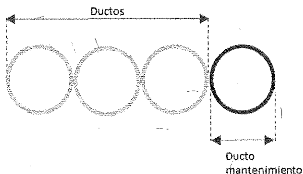
Figura 5. 3 a 7 Ductos, Instalación de Ducto o subducto para mantenimiento.
