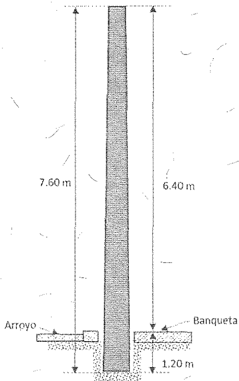
POSTE DE MADERA DE 7.60m
