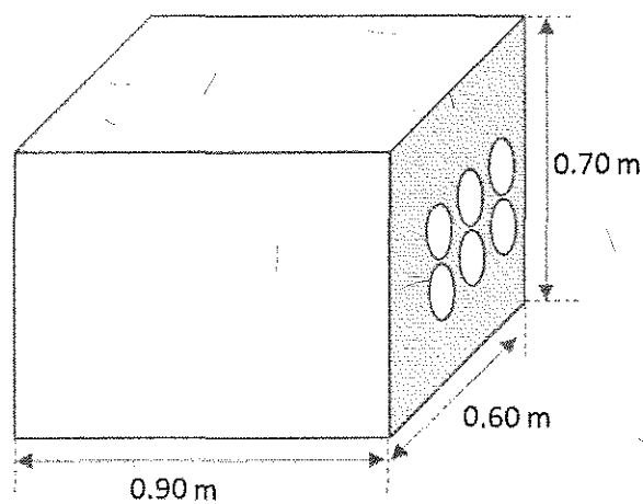
Figura 7. Caja de empalme/registro
