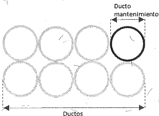
Figura 6. Más de 8 Ductos, Instalación de Ducto para mantenimiento.
