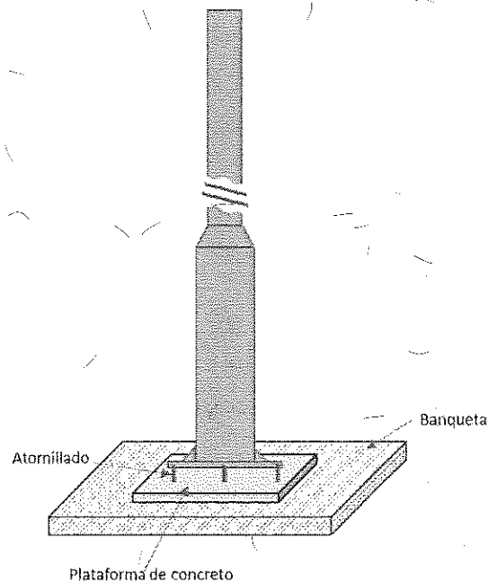
Figura.5 Poste de Acero
