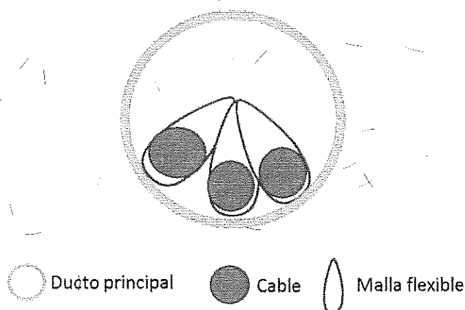
Figura 9. Uso de malla flexible
