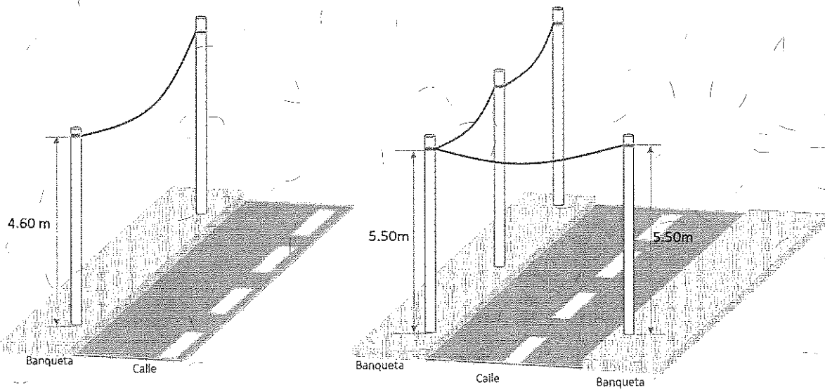
Figura 9. Altura mínima en banqueta y cruce de calle
