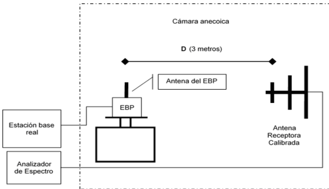
Figura 3. Configuración para medición de emisiones radiadas.
