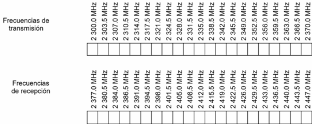
Figura 1. Banda de frecuencias y su canalización.
