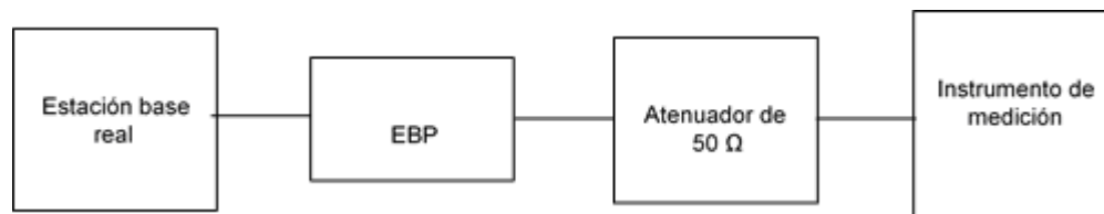
Figura 2. Configuración para medición de emisiones conducidas.
