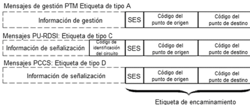
FIGURA 10.- Tipos de etiqueta de mensajes de SS7.
