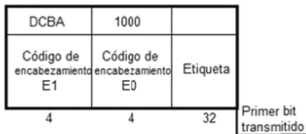
FIGURA 42-A.- Mensaje de acuse de recibo de la conexión de enlace de datos de señalización.
