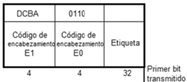
FIGURA 40-A.- Mensaje de inhibición por el sistema de gestión.
