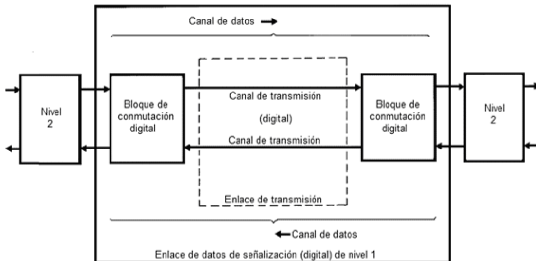
FIGURA 18.- Configuración funcional de un enlace de datos de señalización.
