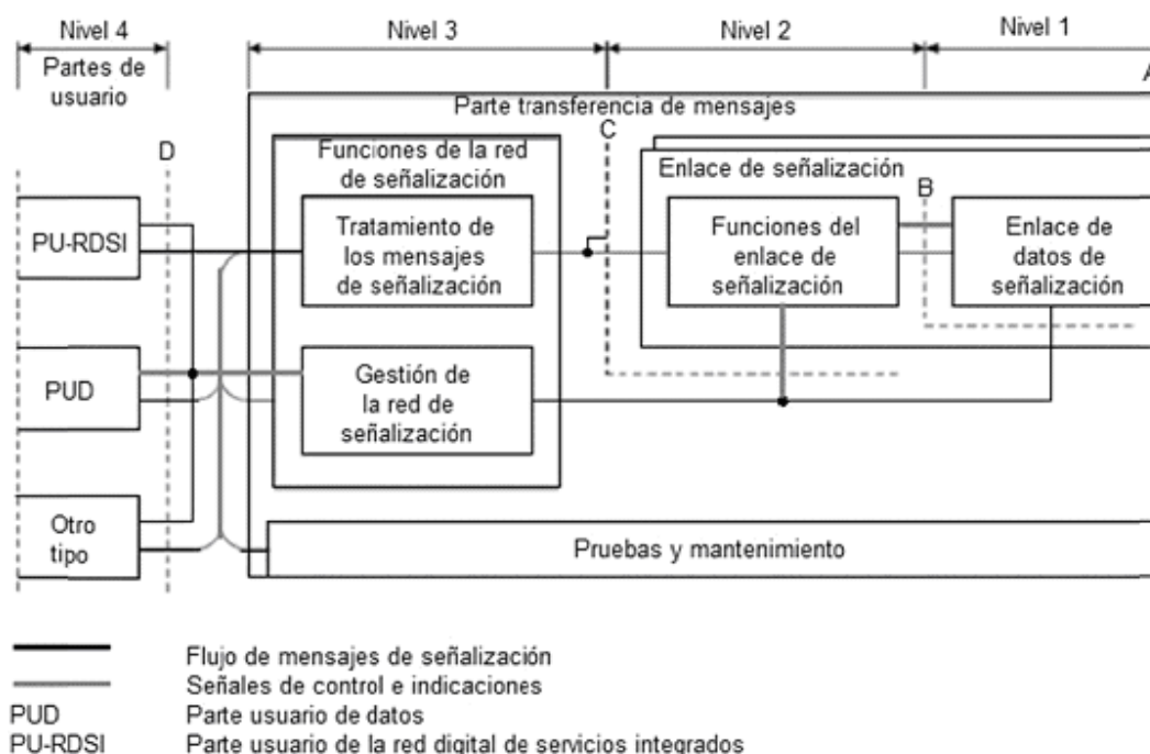
FIGURA 15.- Estructura general de las funciones del sistema de señalización.
