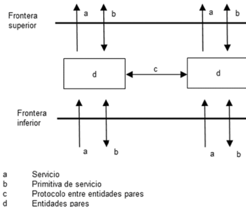
FIGURA 6.- Tipos de primitivas de servicio.
