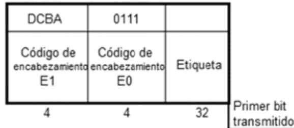
FIGURA 41.- Mensaje de reanudación de tráfico autorizada.
