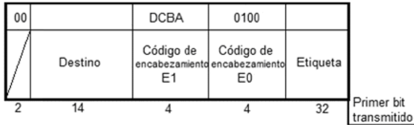
FIGURA 39.- Mensaje de transferencia autorizada.
