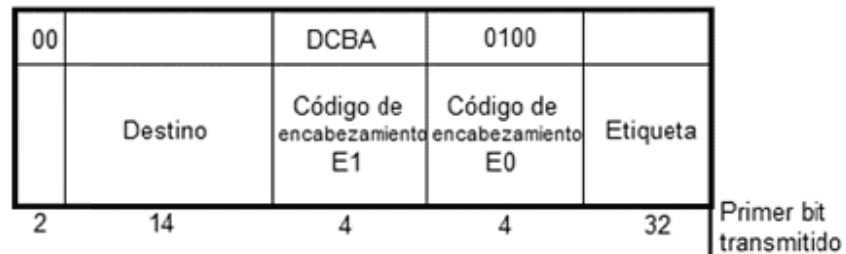
FIGURA 38.- Mensaje de transferencia prohibida.
