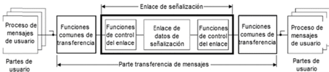
FIGURA 14.- Diagrama funcional del sistema de señalización por canal común.
