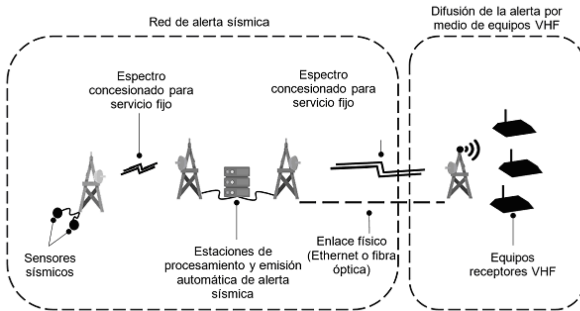
Figura 2. Alternativa de difusión de alerta a equipos receptores en VHF
