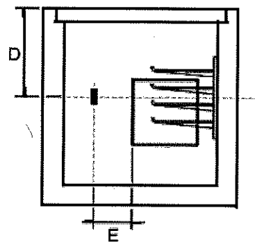
UBICACION DE BASTIDORES Y SOPORTES
