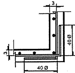
DETALLE TIPO DE ANCLAJES PLANTA O ELEVACIÓN
