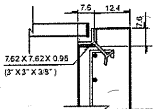
DETALLE TAPA CON REGISTRO
