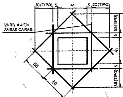
REFUERZO DEL HUECO
