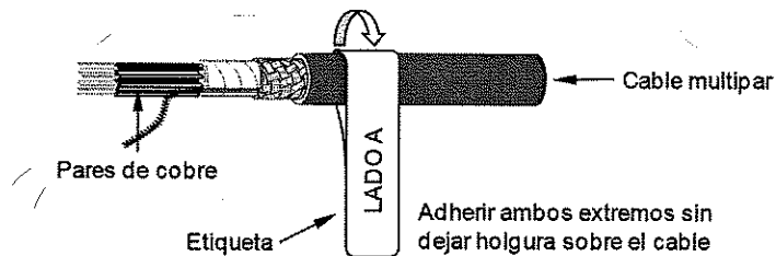
Figura 4.- Ejemplo de colocación de etiqueta para cables multipar.
