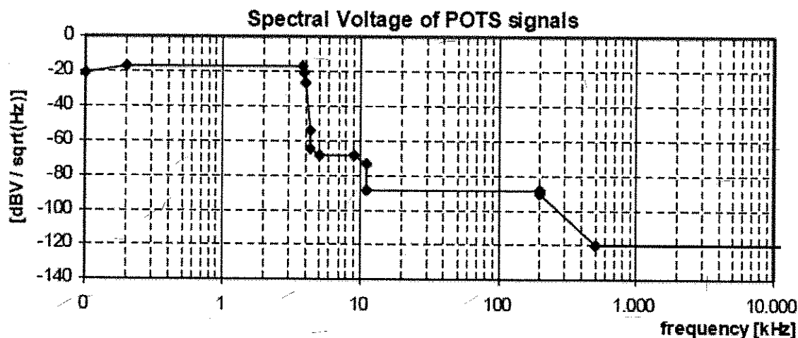
Figura 5 Voltaje espectral para señales POTS.
