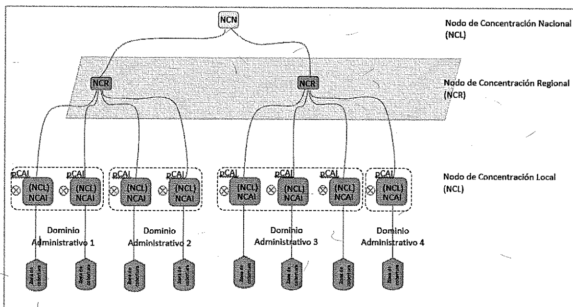
Diagrama de red con los elementos que intervienen en el SCyD 31
