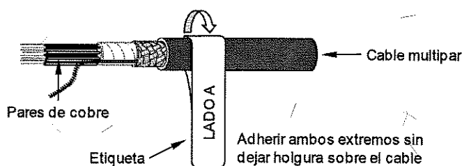
Figura 4.- Ejemplo de colocación de etiqueta para cables multipar.
