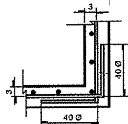
DETALLE TIPO DE ANCLAJES PLANTA O ELEVACIÓN
