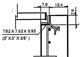
DETALLE TAPA CON REGISTRO
