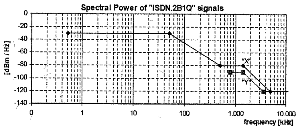
Figura 6 Potencia espectral para señales ISDN 2B1Q.
