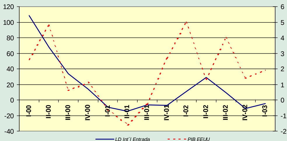
LD Int'l. de Entrada (miles de minutos) vs PIB EEUU: Variación Porcentual Anual
