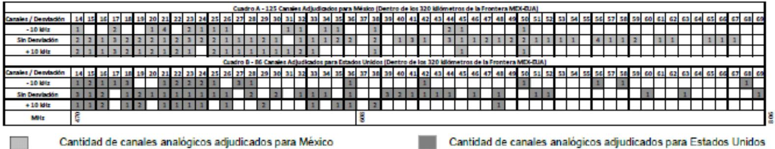
Figura 3. Plan de adjudicación de canales en la banda de UHF entre MEX - EUA
