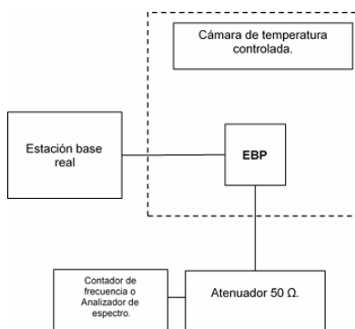
Figura 8. Conexión típica de la instrumentación y EBP para la prueba de Tolerancia en frecuencia.
