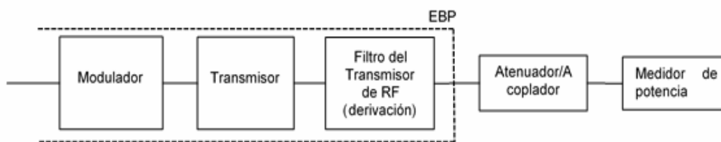
Figura 6. Configuración de prueba conducida para la potencia media de RF.
