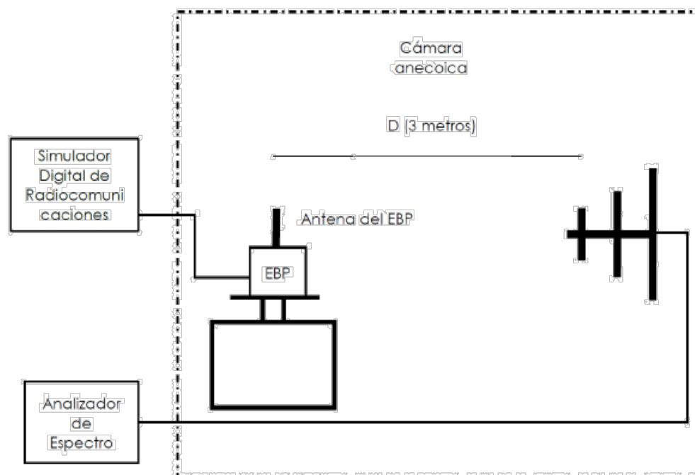
Figura 2. . Configuración para medición de emisiones radiadas
