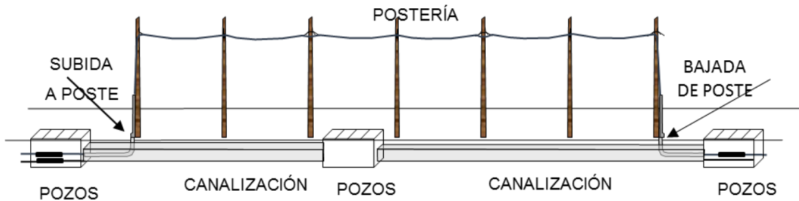
Figura 2. Obra civil
