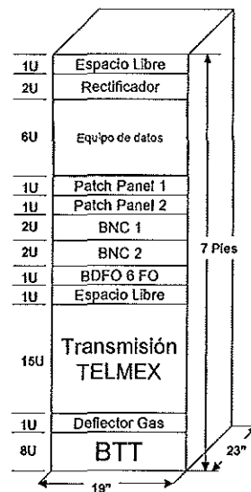
Distribución del gabinete universal Telmex
