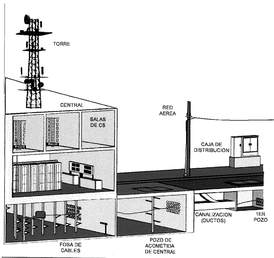
Figura 4. Tendido de Cable sobre Infraestructura Desagregada.
