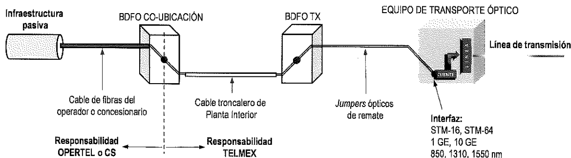
Figura 4 Conexión del servicio de canal óptico.
