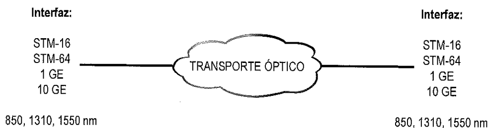
Figura 3 Arquitectura del servicio de canal óptico.
