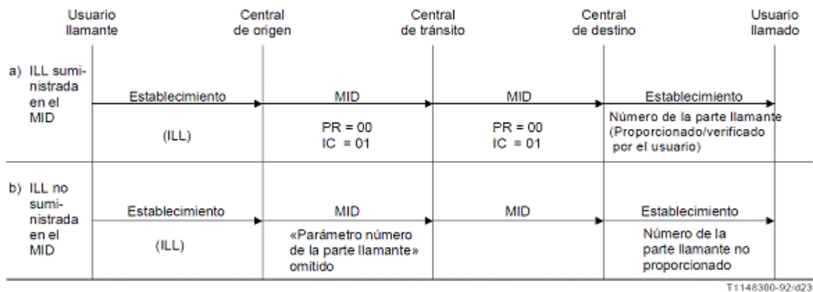
FIGURA 51.- Presentación de la identificación de la línea llamante. Presentación permitida - ILL proporcionada por el usuario llamante.
