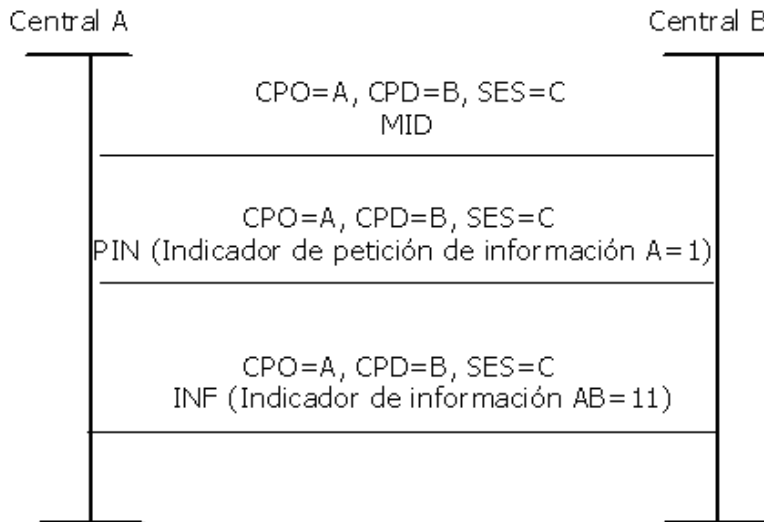
FIGURA 42.- Secuencia de los mensajes de información.
