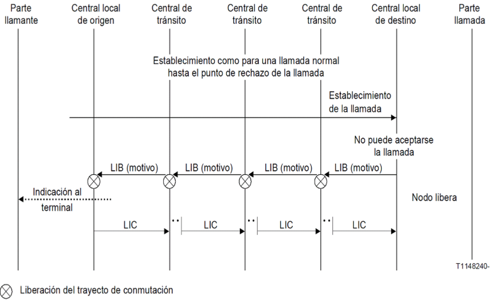
FIGURA 45.- Establecimiento de llamada no completado (no hay reencaminamiento).
