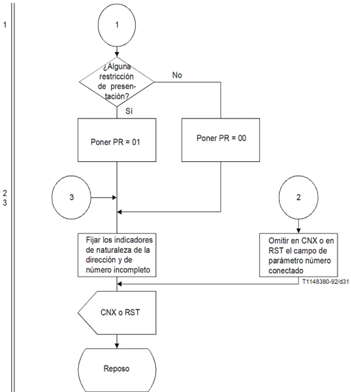
FIGURA 58 (hoja 1 de 2).- Funciones de señalización nodal de central local de destino para PILC y RILC. (Esta figura no es aplicable al interfaz y se da únicamente a título informativo).
