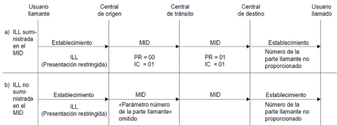
FIGURA 53.- Restricción de identificación de la línea llamante. Presentación no permitida - ILL proporcionada por la central de origen.
