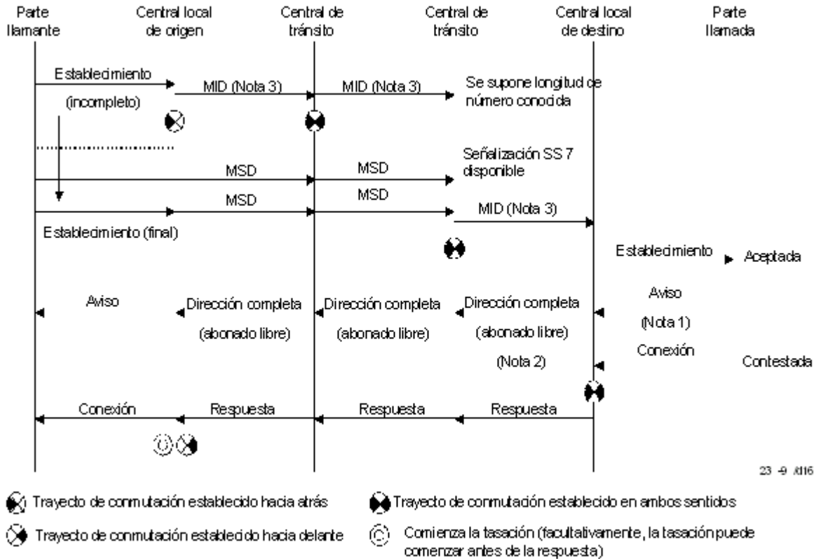
FIGURA D-2/Q.767
