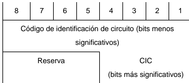
FIGURA 2.- Campo de identificación de circuito.
