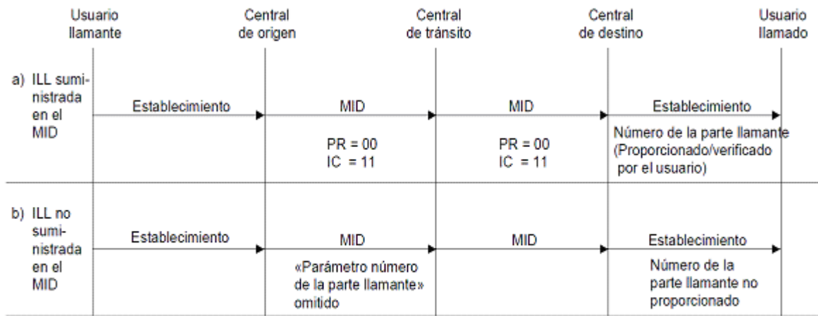
FIGURA 51.- Presentación de la identificación de la línea llamante. Presentación permitida - ILL proporcionada por el usuario llamante.
