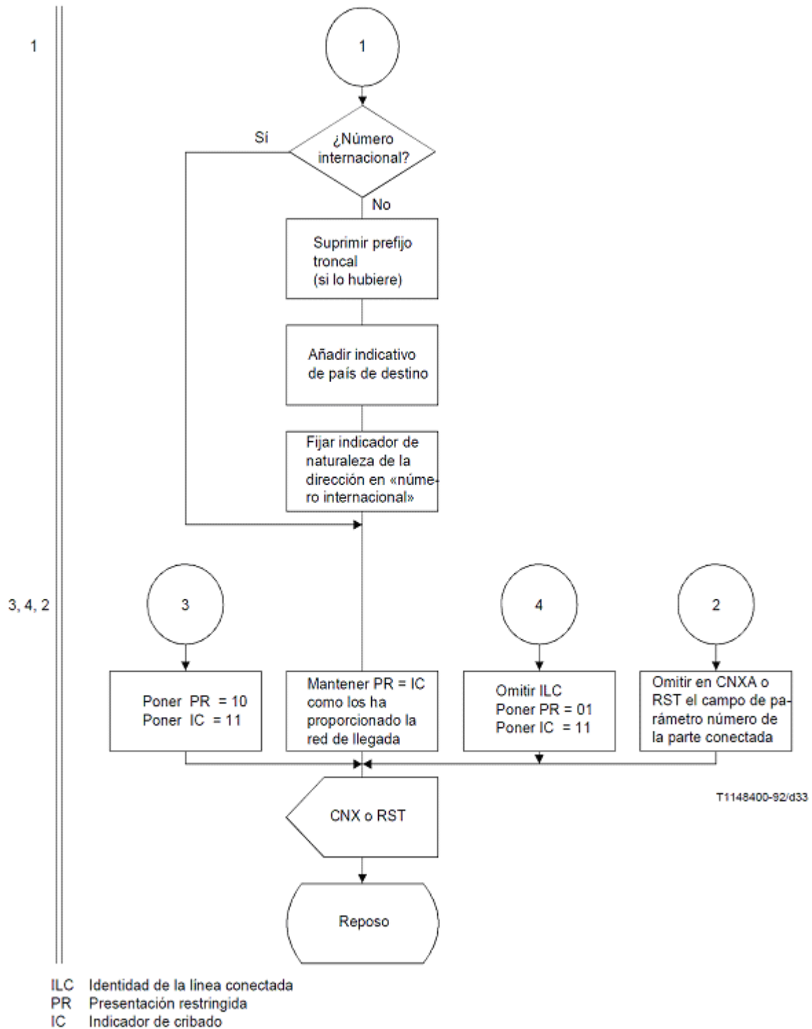
FIGURA 59 (hoja 2 de 2).- Funciones de señalización nodal de cabecera internacional de llegada para PILC y RILC.
