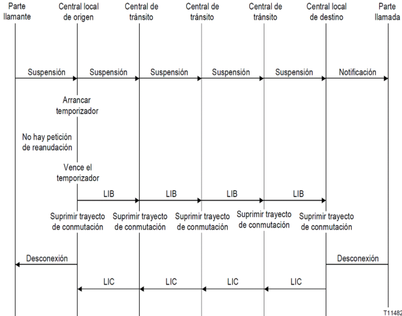
FIGURA 47.- Petición de suspensión sin conexión.
