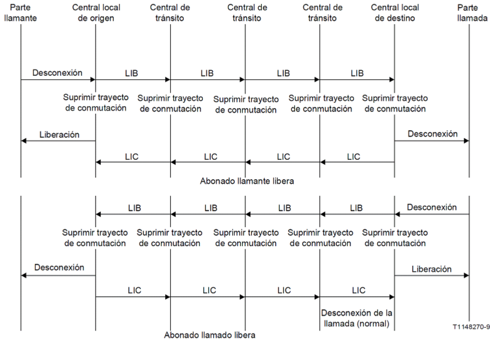
FIGURA 48.- Liberación de llamada normal.
