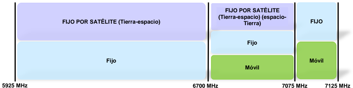
Imagen 1. Representación gráfica de la atribución nacional de la banda de frecuencias 5925-7125 MHz
