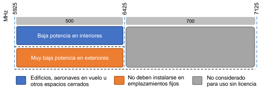
Imagen 10. Representación gráfica del uso sin licencia en la banda de frecuencias 5925-7125 MHz en Reino Unido
