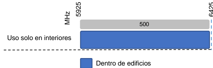
Imagen 11. Representación gráfica del uso sin licencia recomendado en la banda de frecuencias 5925-7125 MHz en la Unión Europea
