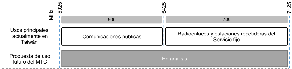
Imagen 9. Representación gráfica del uso de la banda de frecuencias 5925-7125 MHz en Taiwán
