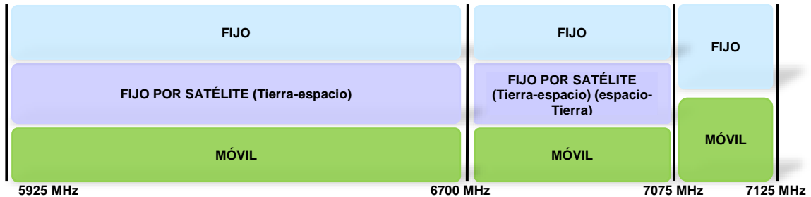
Imagen 3. Representación gráfica de la atribución internacional de la banda de frecuencias 5925-7125 MHz
