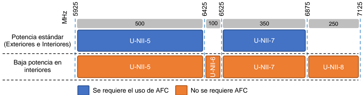
Imagen 4. Representación gráfica del uso sin licencia en la banda de frecuencias 5925-7125 MHz en EUA
