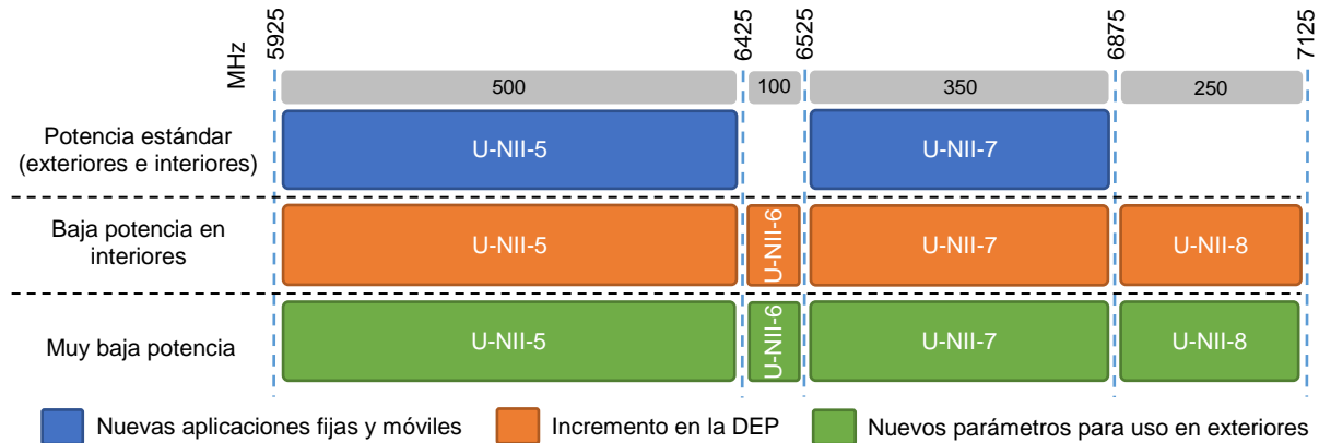
Imagen 5. Representación gráfica de posibles consideraciones en la banda de frecuencias 5925-7125 MHz en EUA
