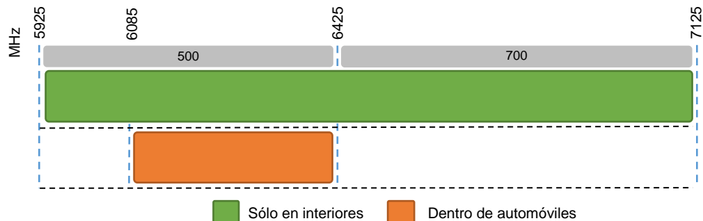
Imagen 8. Representación gráfica del uso sin licencia propuesto para la banda de frecuencias 5925-7125 MHz en Corea del Sur
