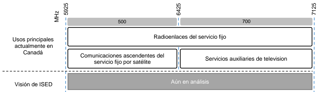
Imagen 6. Representación gráfica del uso de la banda de frecuencias 5925-7125 MHz en Canadá
