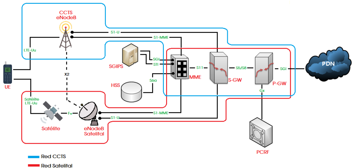
Figura 2. Elementos mínimos y arquitectura de la red para el Servicio Complementario Terrestre del Servicio Móvil por Satélite
