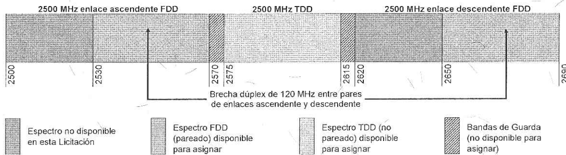
Figura 2: Banda de 2500 MHz en México.
