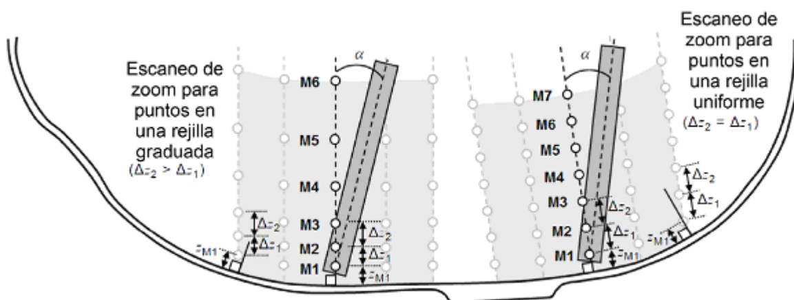
Figura 11. Orientación de la sonda con respecto a la línea normal a la superficie del MAC, mostrada en dos ubicaciones diferentes.
