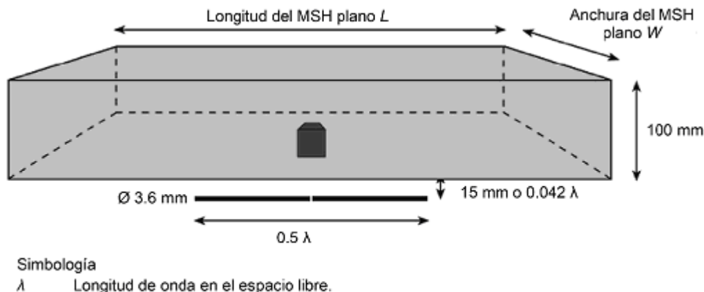
Figura S.2. Dimensiones del MSH plano con un cubo de 10 g mostrado en el centro del mismo.
