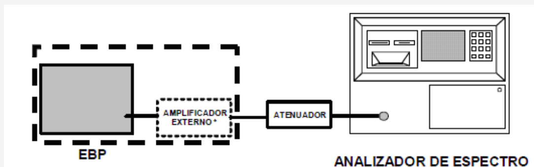
Figura 1 Configuración para medición de emisiones conducidas
