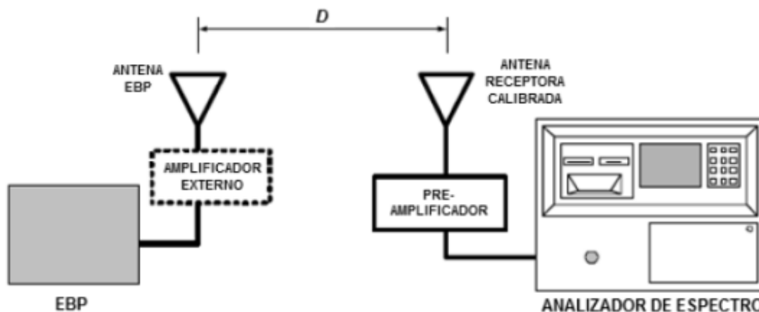
Figura 2. Configuración para medición de emisiones radiadas.
