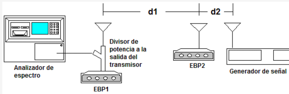
Figura 3 Configuración de prueba de existencia de inteligencia para reconocer canales de posición de frecuencia ocupados
